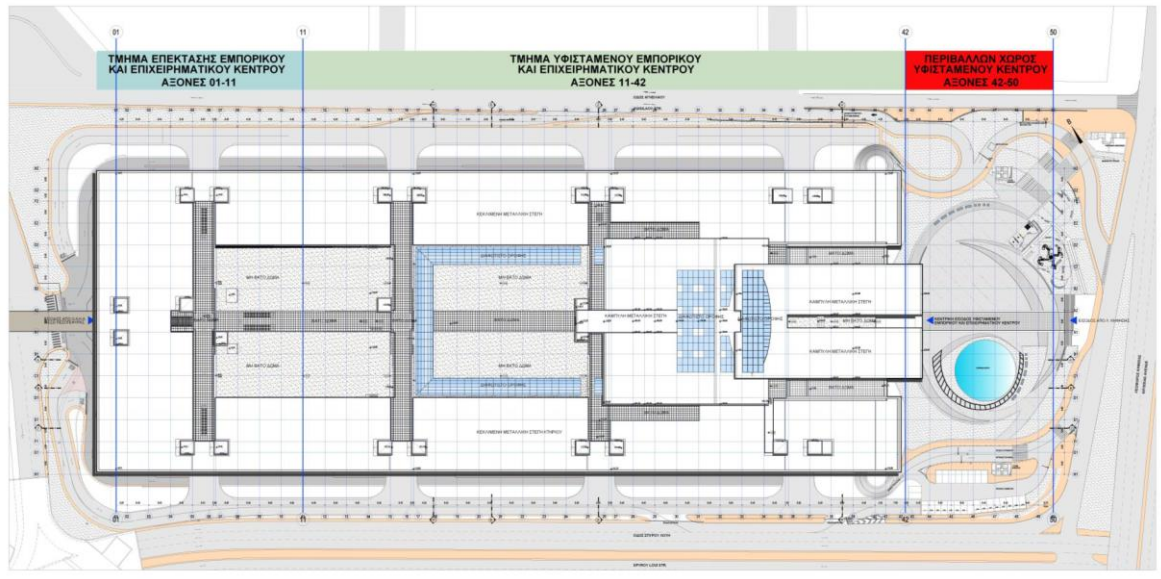
Σχήμα 1: Κάτοψη Κτιρίου
